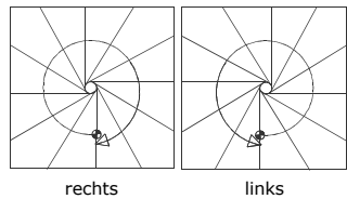
13 Steigungen
